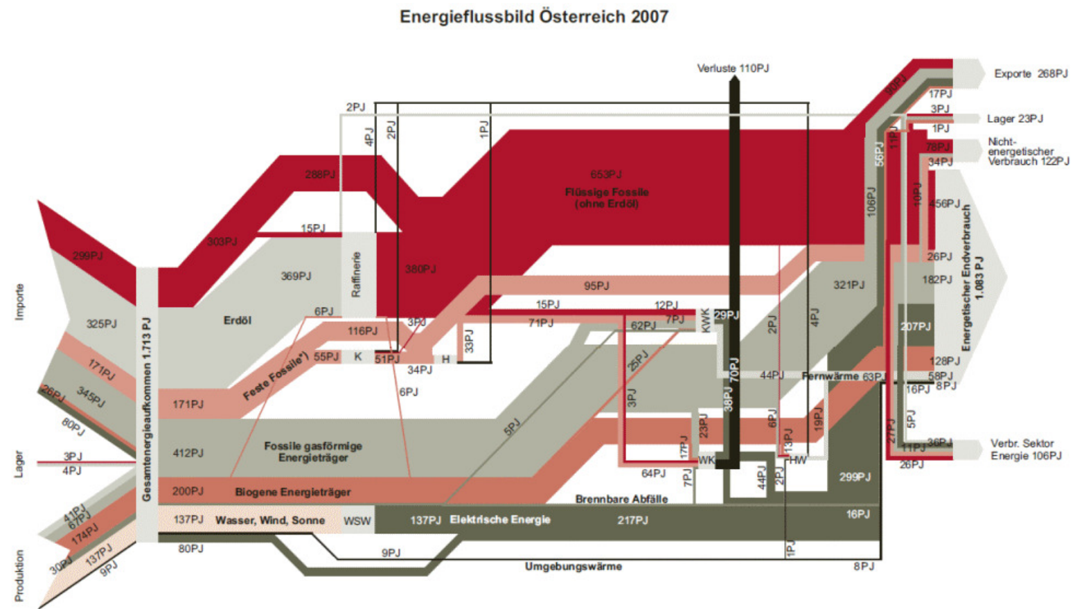
Abbildung 13: Energieflussdiagramm
