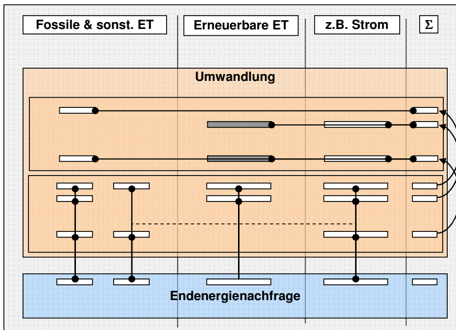
Abbildung 18: Energieumwandlung
