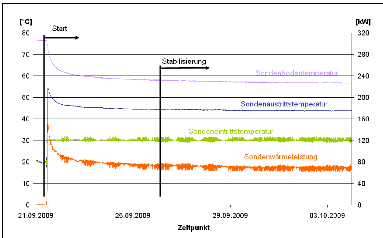
Abbildung 8: Temperatur- & Leistungsverhalten
