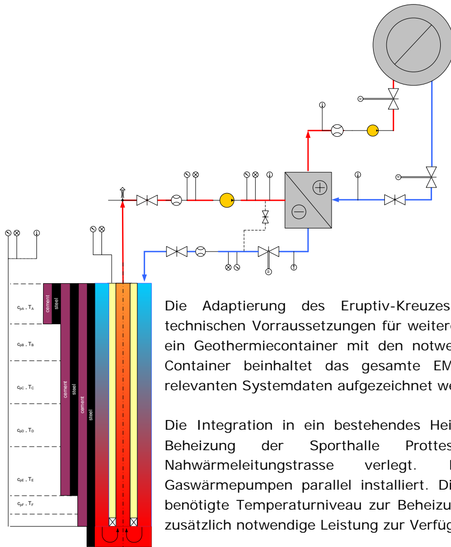
Abbildung 1: Funktionschema
