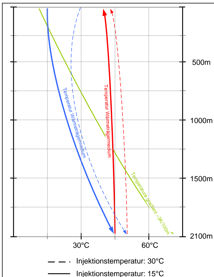
Abbildung 3: Temperaturverlauf
