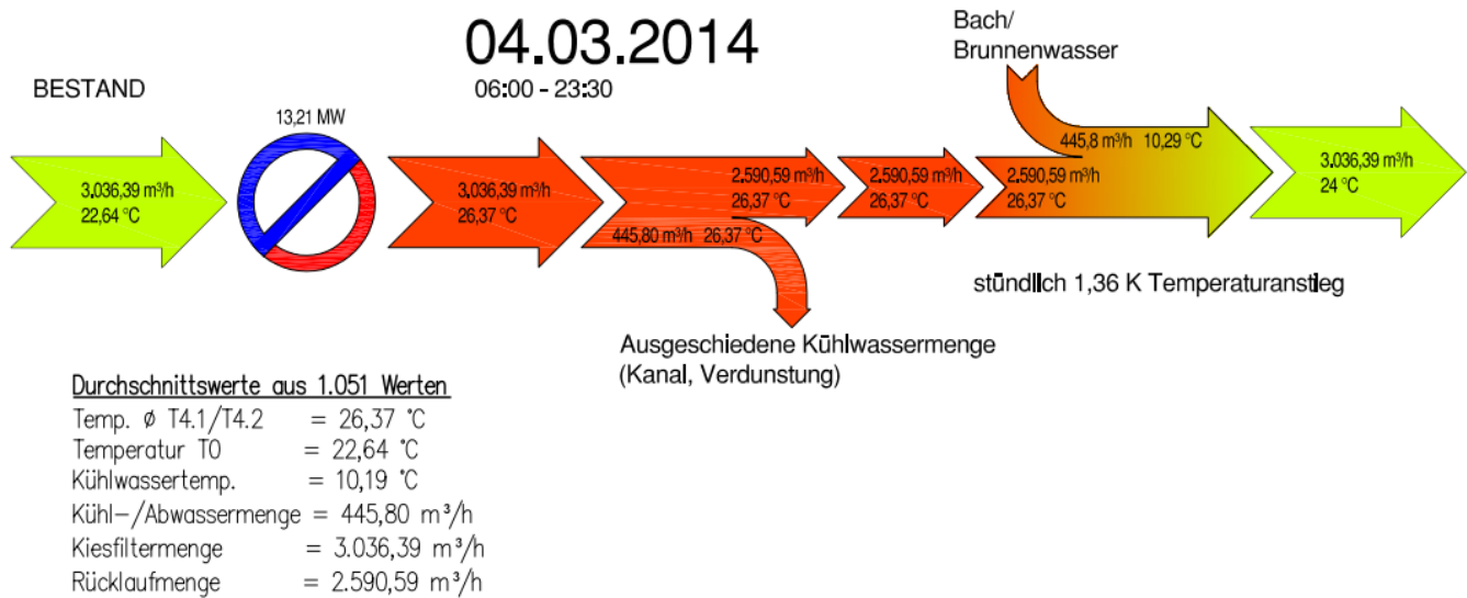
Abbildung 15: Temperaturanstieg 04.03.2014 4
